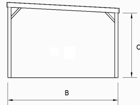
Façade latérale droite
