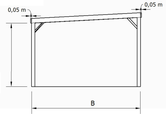
Façade latérale gauche
